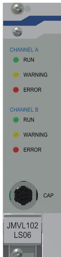
Obr. 27: Příklad čelního panelu jednotky LS06
