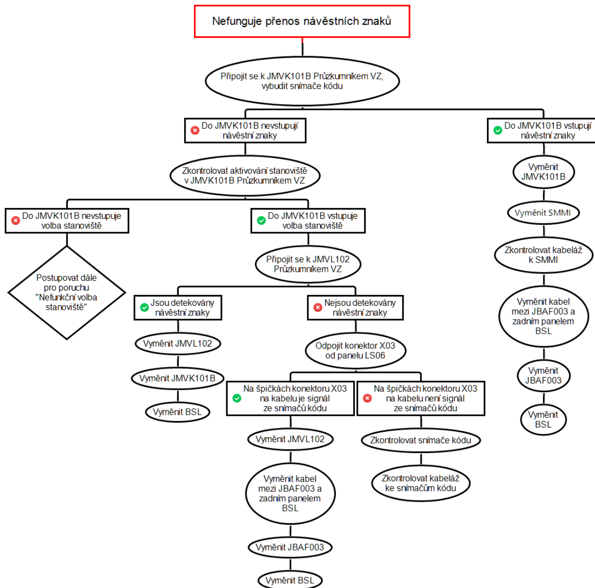
Obr. 7: Lokalizace vadného dílu při poruše Nefunkční přenos návěstních znaků
