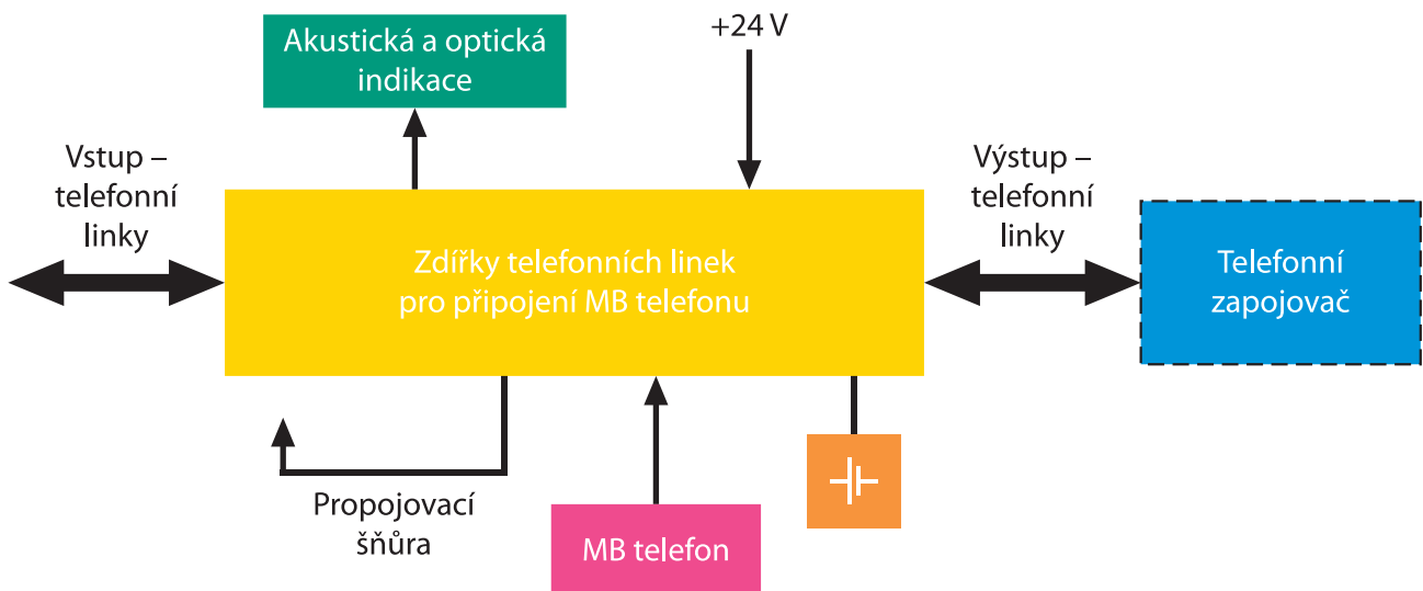
Blokové schéma
