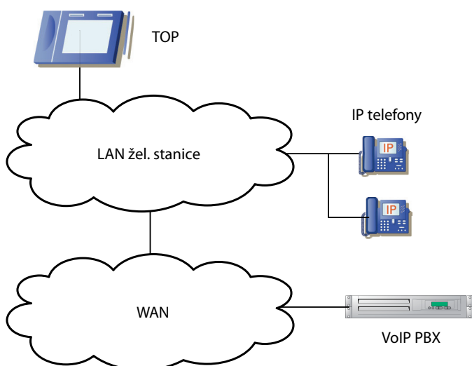
Schéma propojení ústředny s okolím
